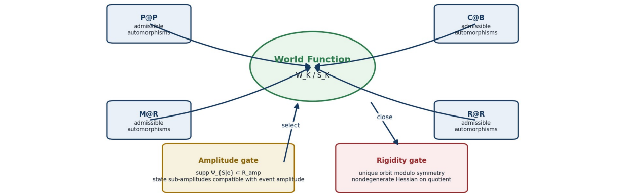
Рисунок П.2. Пакетная ковариантность, согласование амплитуд и финальная жёсткость.
