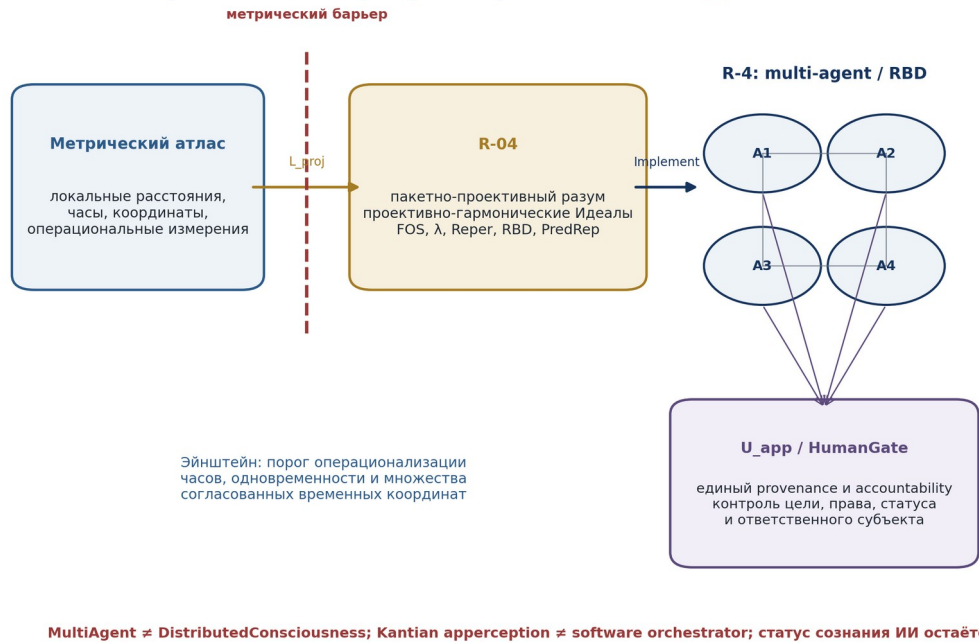
Рисунок 12.4. R–04/R–4: метрический барьер, проективные Идеалы, многоагентная реализация и HumanGate.
