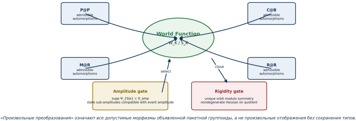
Рисунок П.2. Пакетная ковариантность, согласование амплитуд и финальная жёсткость.
