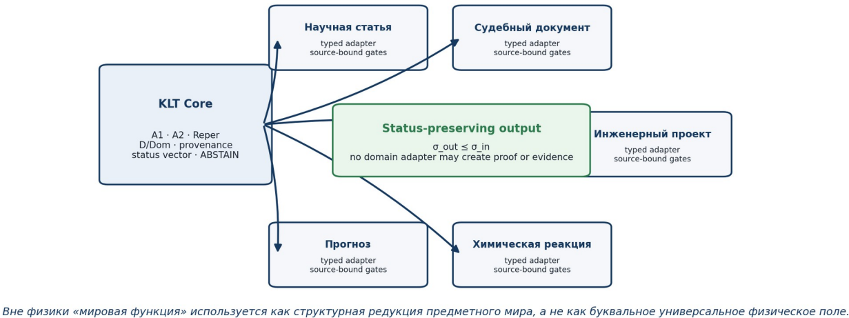
Рисунок 22. Пять предметных адаптеров KLT-RBD и общий status-preserving output.
