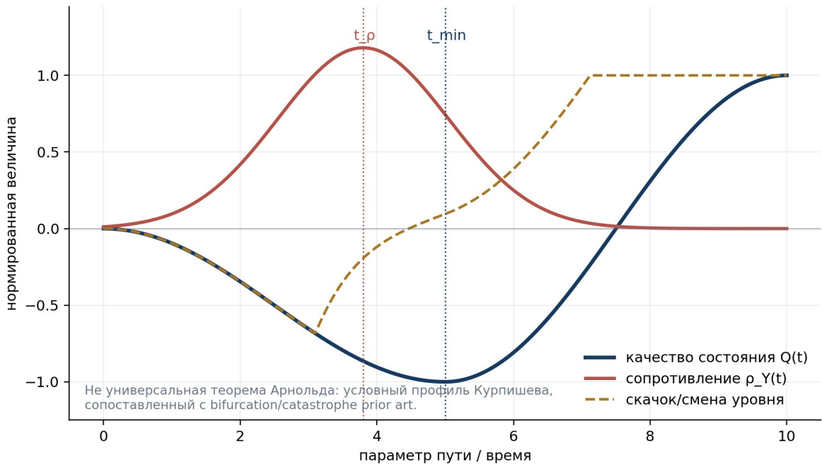
Рисунок 8. KLT-профиль АК-6 на основе A6_Arnold: равенство амплитуд и лабиринт показаны только как отдельные расширения.
