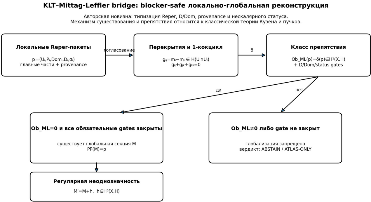
Рисунок 12. Пучковая глобализация отделена от KLT-гейтов: кохомологическое препятствие отвечает за математическое существование, а D/Dom/provenance/status — за разрешённость вывода в проекте.
