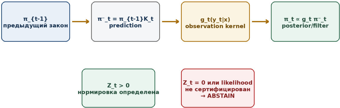
Рисунок 3. Prediction-update цикл и zero-evidence gate.
