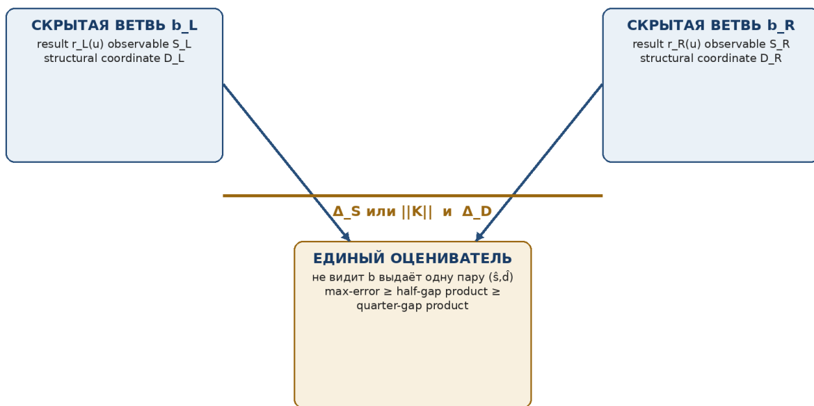
Рисунок 1. Геометрическое ядро локальной минимаксной ПН.2.
