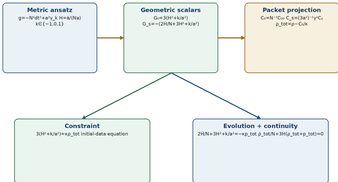
Рисунок 3. Геометрическая скаляризация и packet-corrected bookkeeping.
